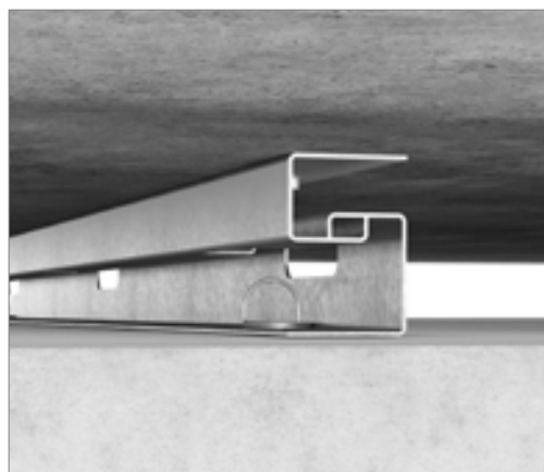
Direktbefestigungsschiene
